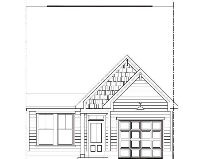
ELEVATION E
